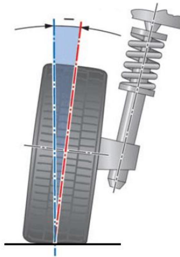
Отрицательный угол развала
