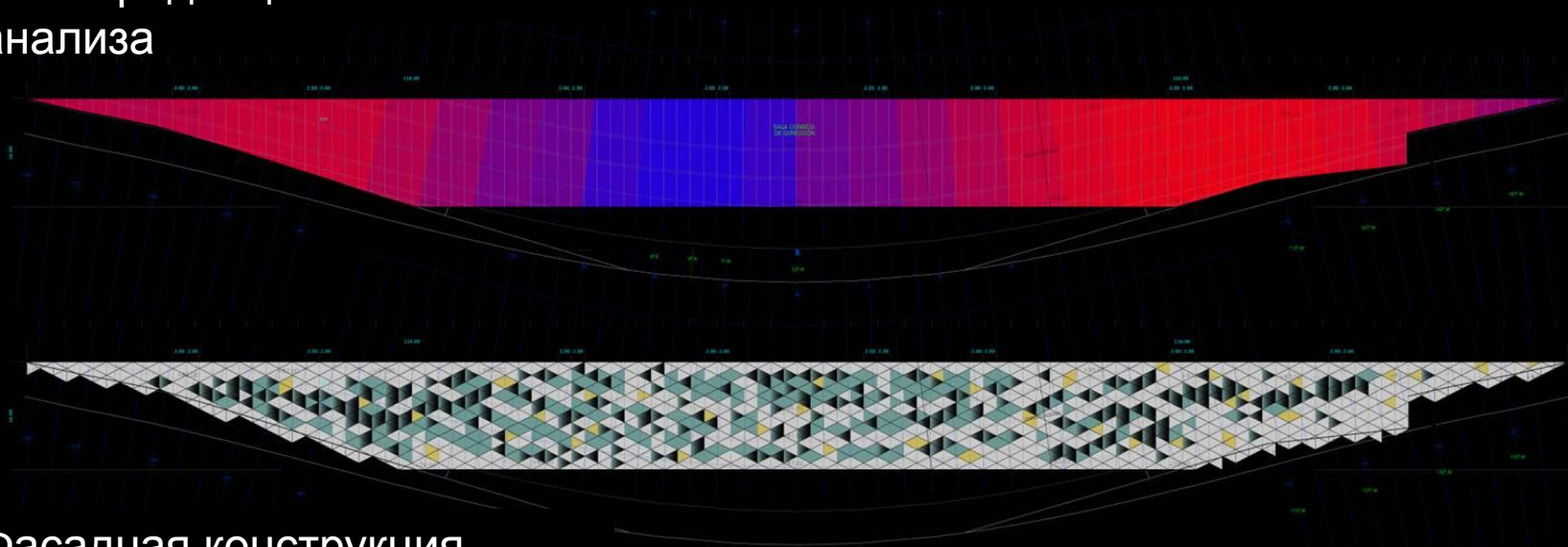
Фасадная конструкция
