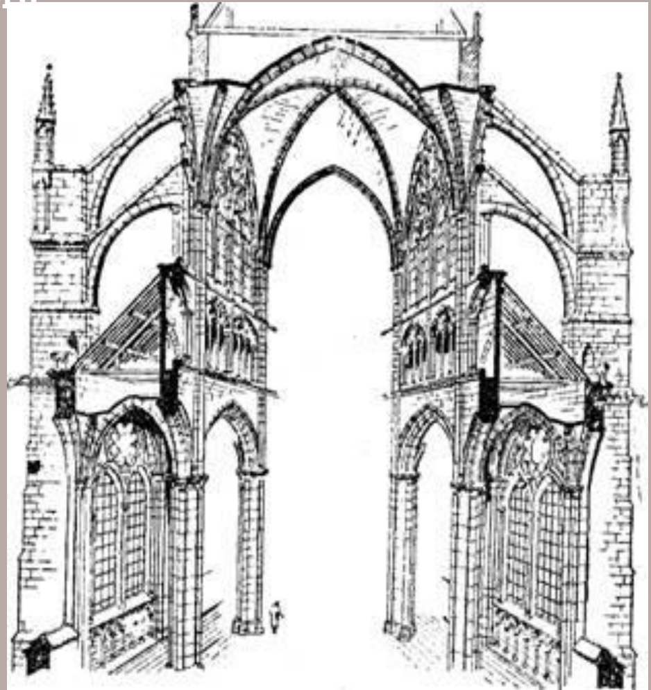
Поперечный разрез готического собора
