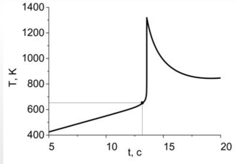
Термограма ТВ
