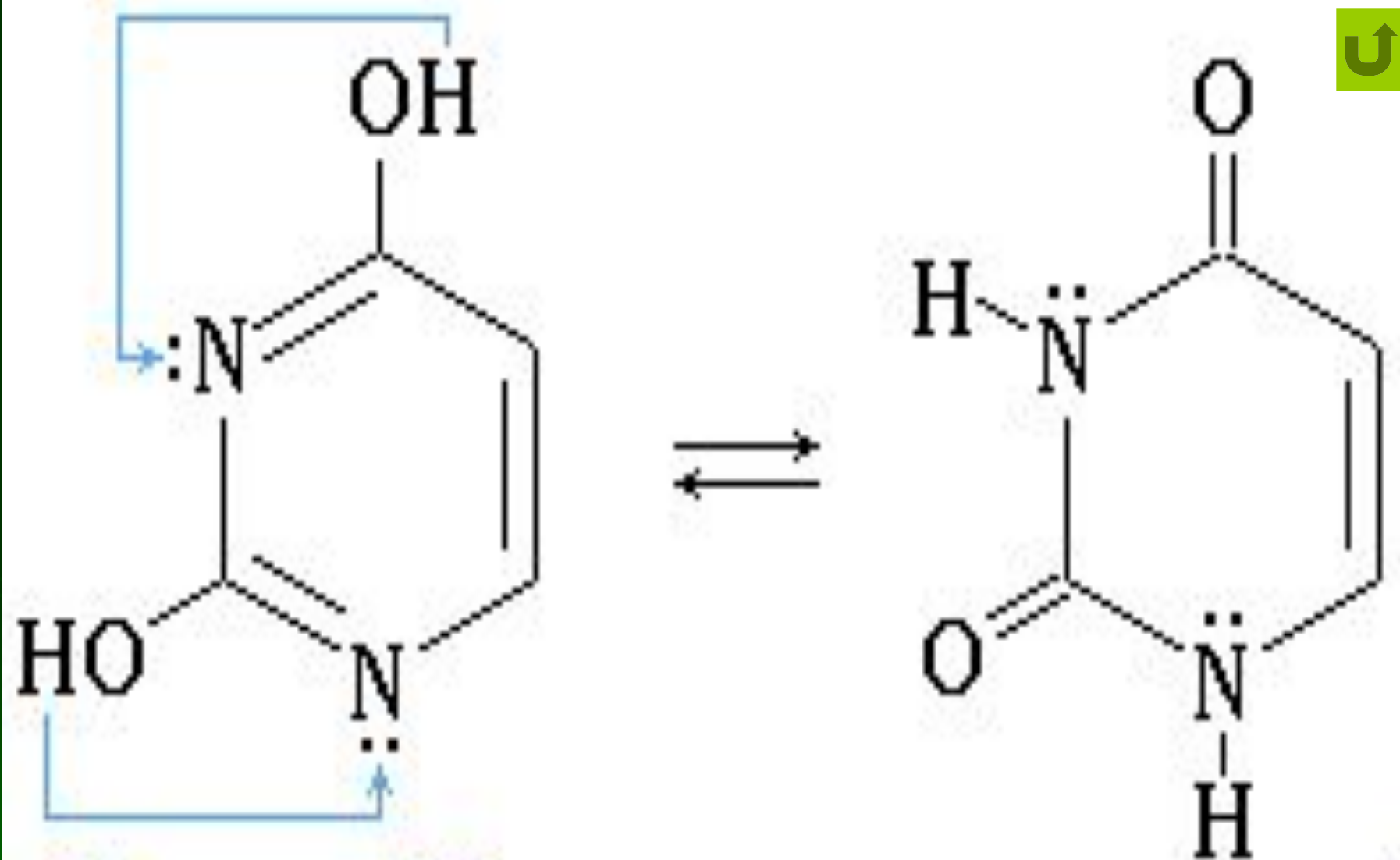
Урацил (2,4-дигидроксиимидин)
