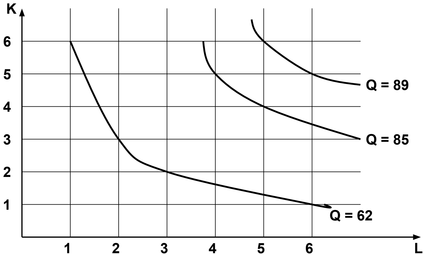
Карта изоквант
