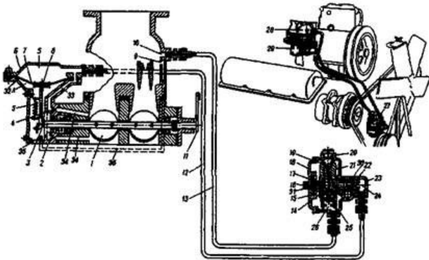
Мал.7.3 Схема обмежувача максимальної частоти обертання колінчастого вала двигуна
