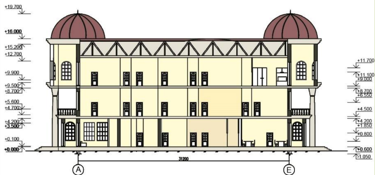
Разрез Б-Б М1:100
