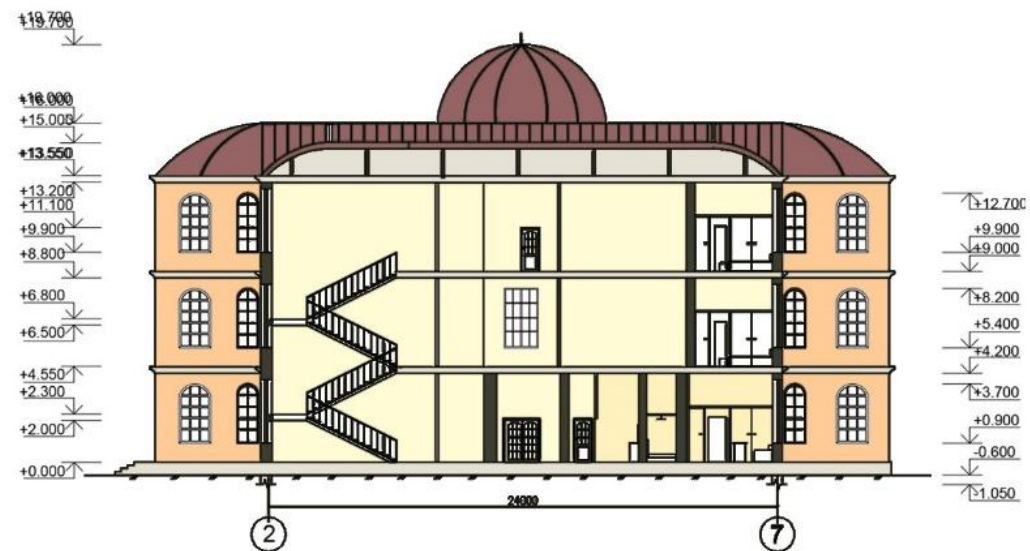
Разрез Б-Б М1:100
