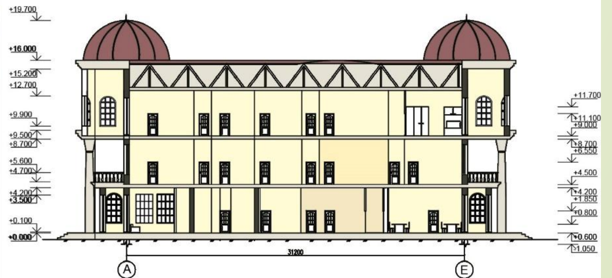
Разрез Б-Б М1:100
