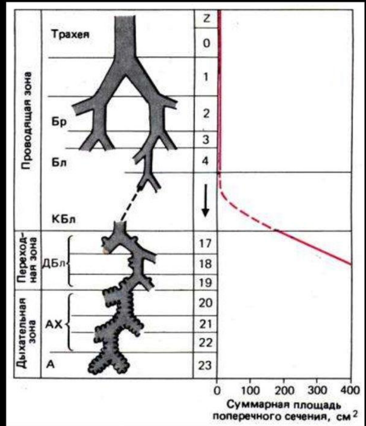
Схема ветвления воздухоносных путей (слева) и кривая суммарной площади поперечного сечения воздухоносных путей на уровне каждого ветвления (справа)
