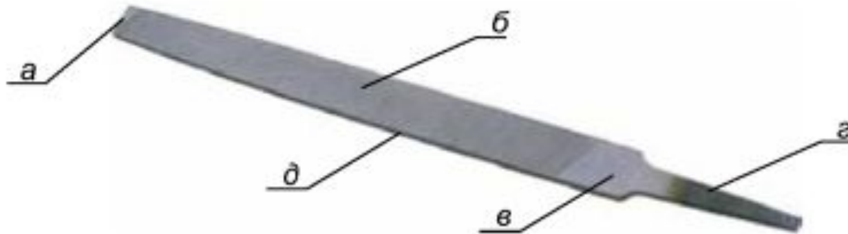
Мал. 88. Будова напилка: а – носок; б – робоча грань; в – п'ятка; г – хвостовик; д – ребро
