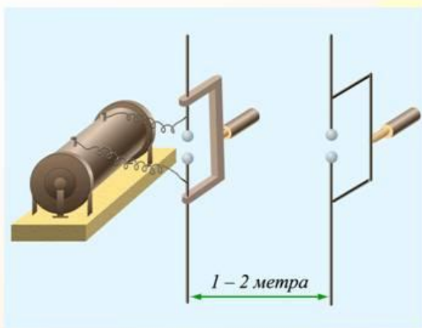
генератор Герца
