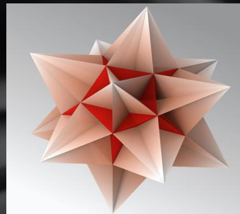
большой икосаэдр
