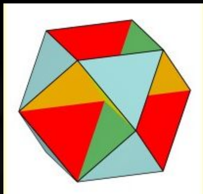
большой додекаэдр
