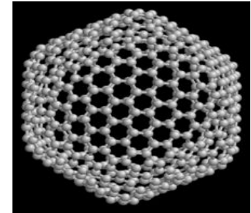
Фуллерен C540
