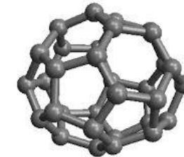
Фуллерен C32
