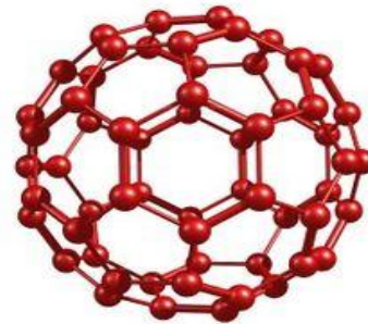
Фуллерен C60
