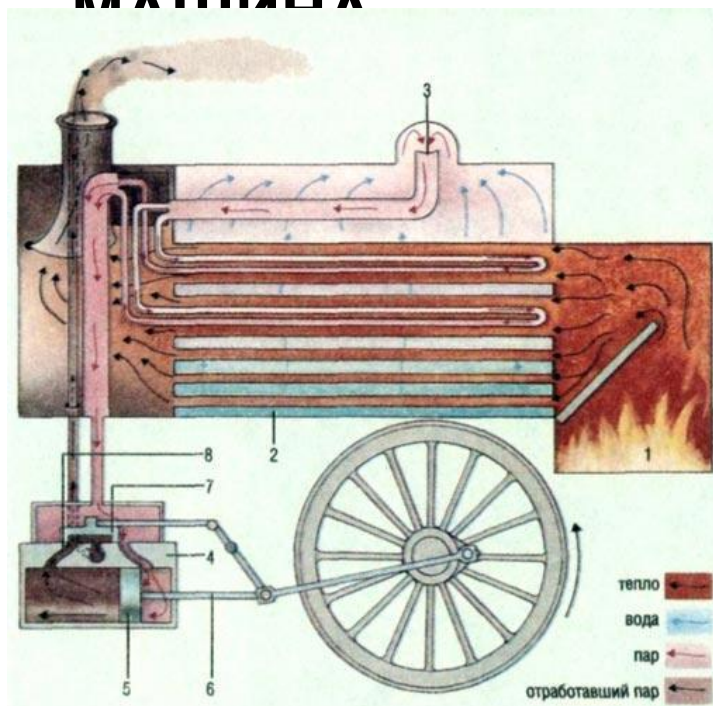
ПАРОВАЯ МАШИНА
