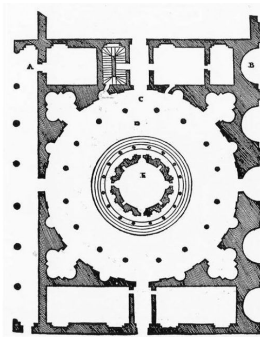
Браманте. Темплетто. 1502
