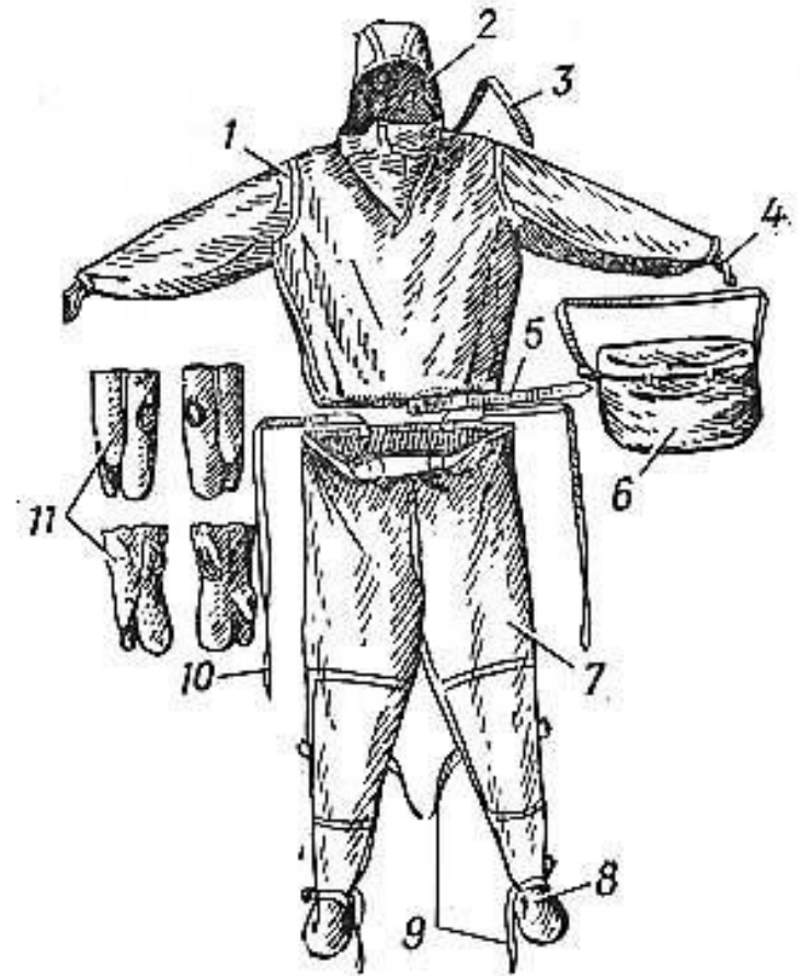
Рис. 6.11. Легкий защитный костюм: 1 — куртка; 2 — капюшон; 3 — горловой хлястик; 4 — петля; 5 — промежуточный хлястик; 6 — сумка; 7 — брюки; 8 — боты; 9 — хлястики; 10 — бретели; 11 — перчатки
