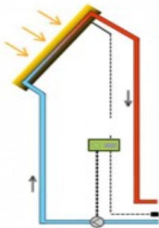
Солнечно-водяной коллектор
