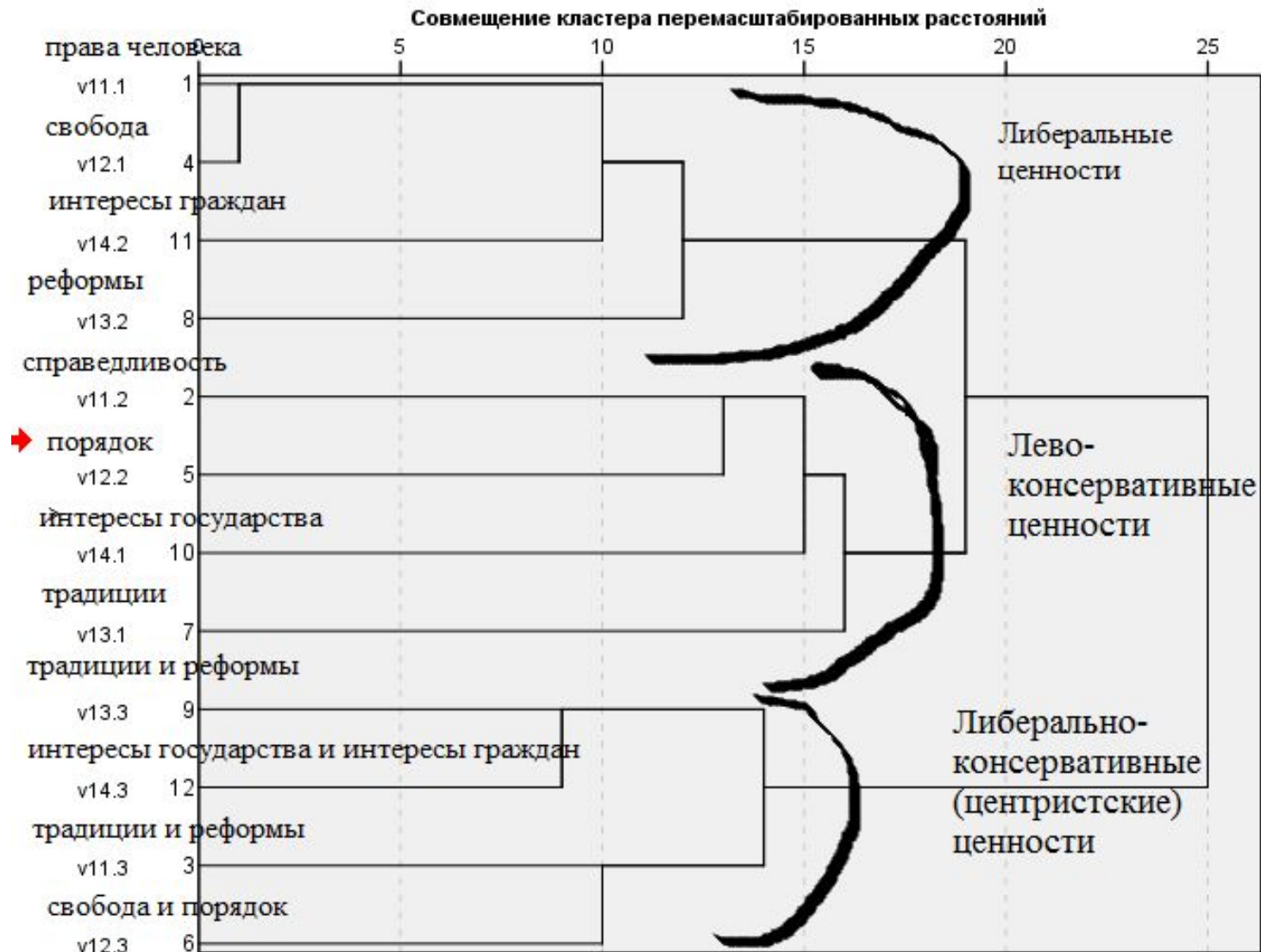
Дендрограмма с использованием метода межгрупповых связей
