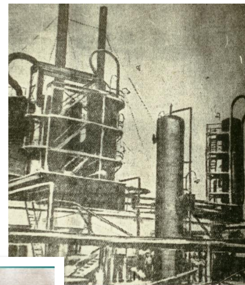
Крекинг-установка 1935г.
