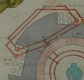
СХЕМА СОЕДИНЕНИЯ ЯКОРА И КОЛЛЕКТОРА ГЕНЕРАТОРА
