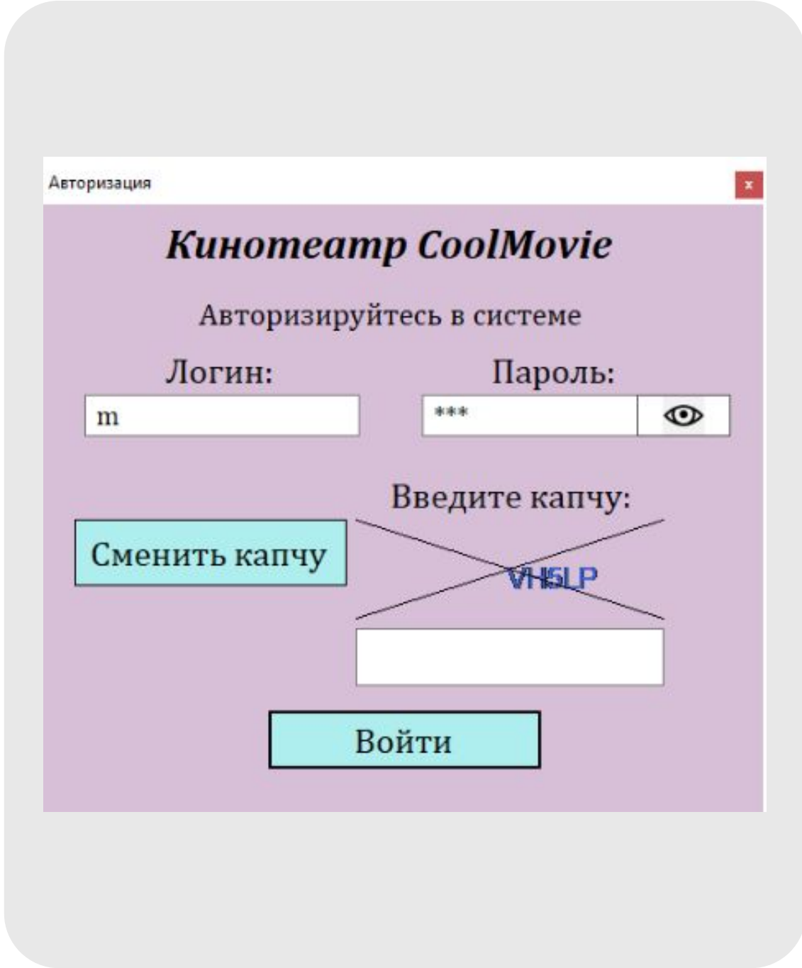
Капча
