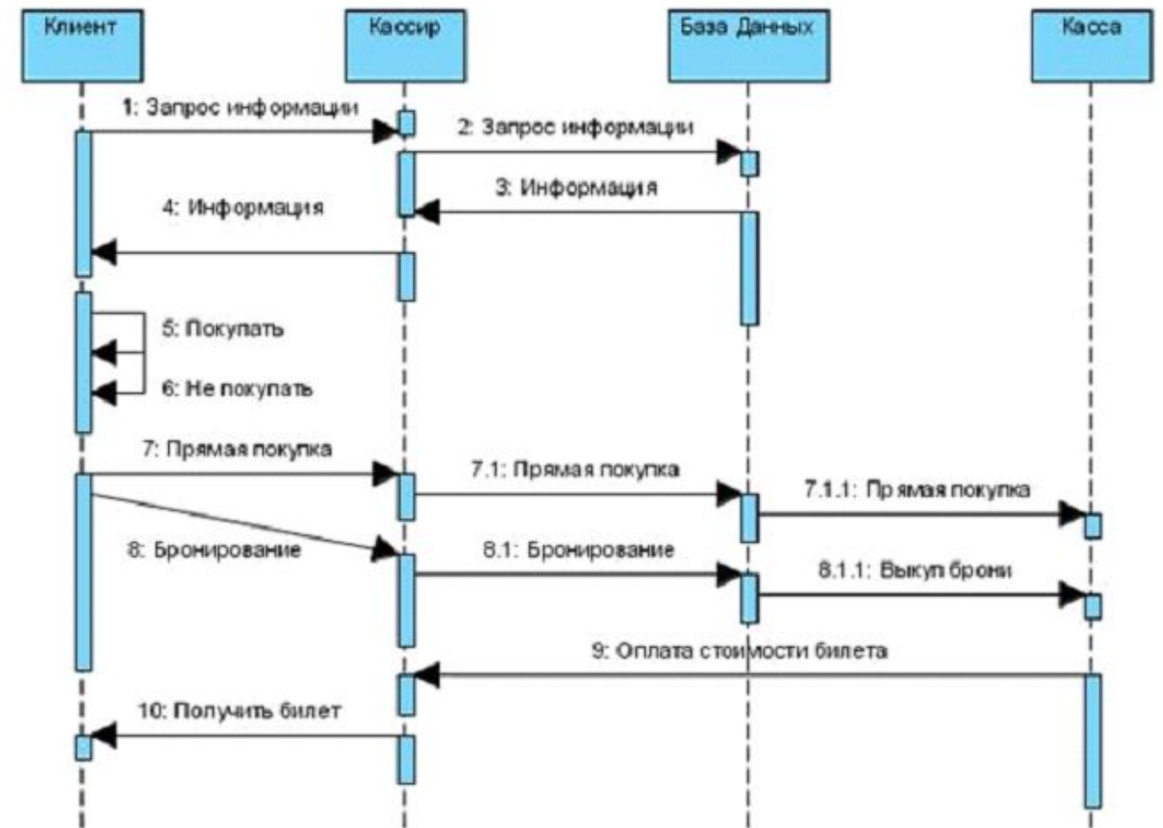
Диаграмма последовательностей
