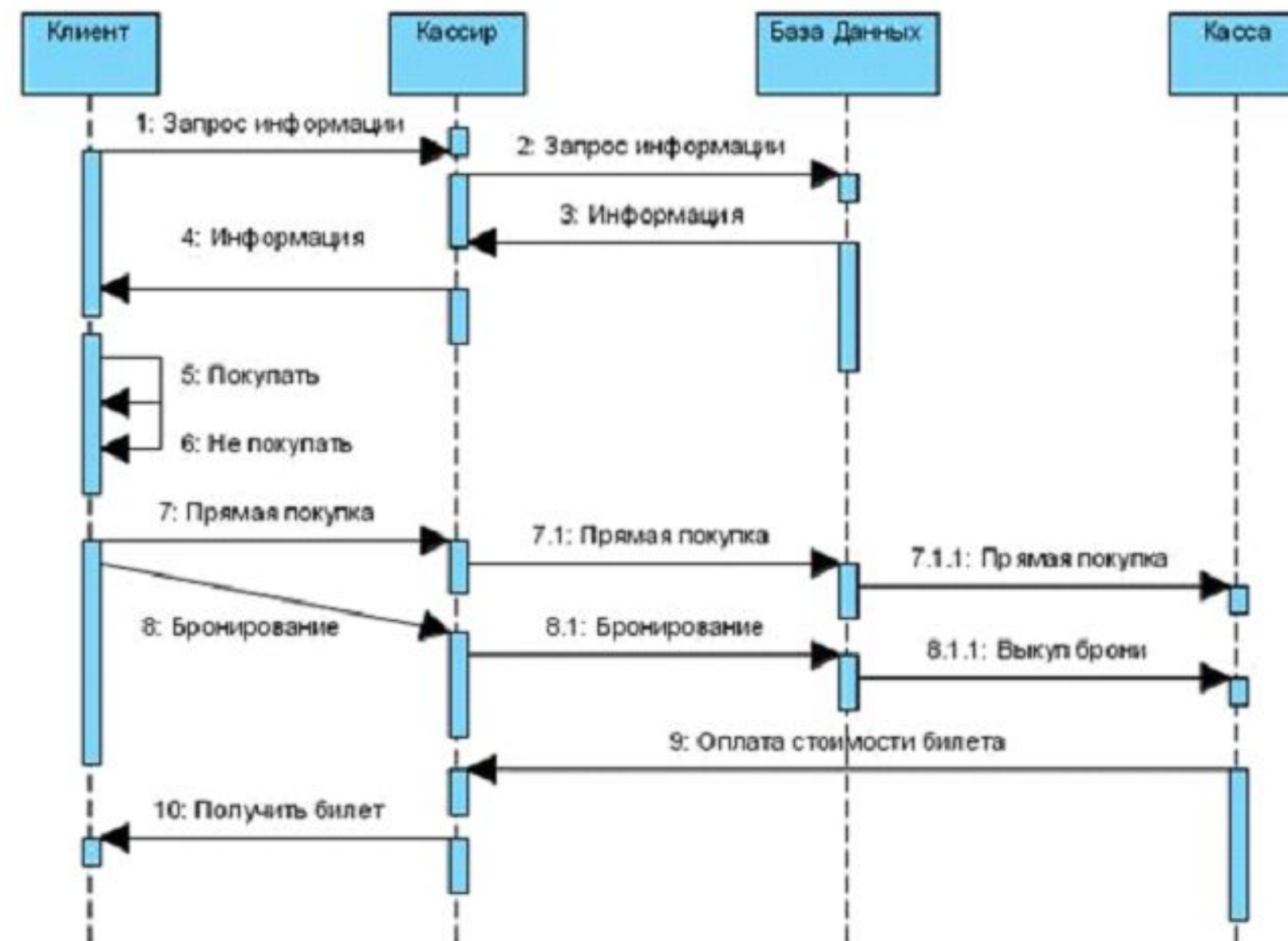
Диаграмма последовательностей
