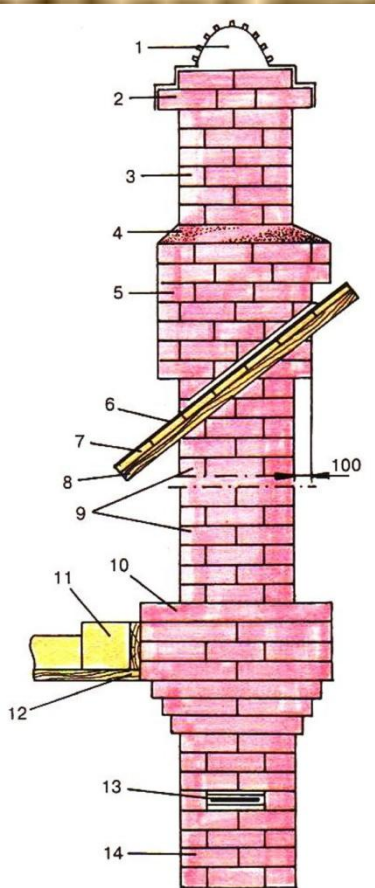
Рис. . Труба и ее части:
