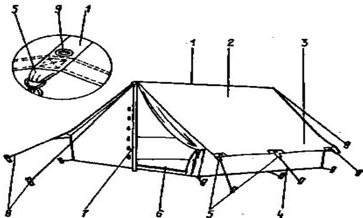
Рис. 4. Туристическая палатка: 1 — конек, 2 — боковой скат, 3 — крыло, 4 — боковая стенка, 5 — проушины, 6 — пол, 7 — опорная стойка, 8 — оттяжки, 9 — люверс.
