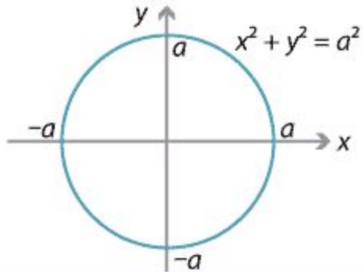
Circle
