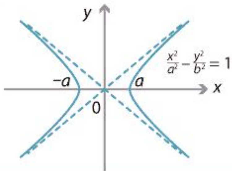
Hyperbola
