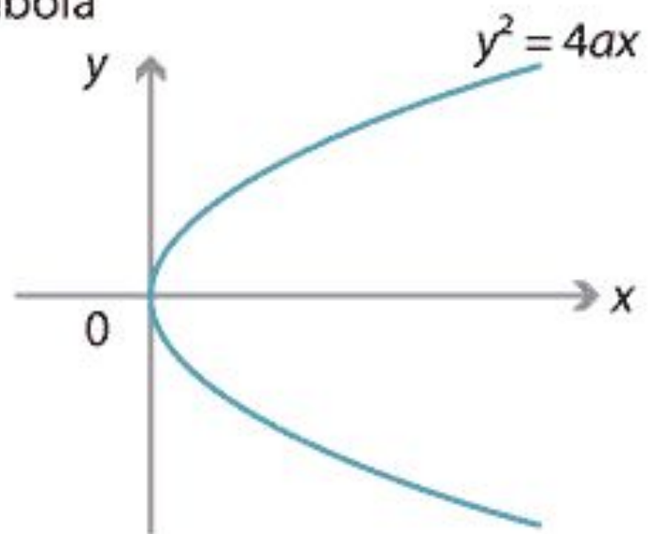
Parabola
