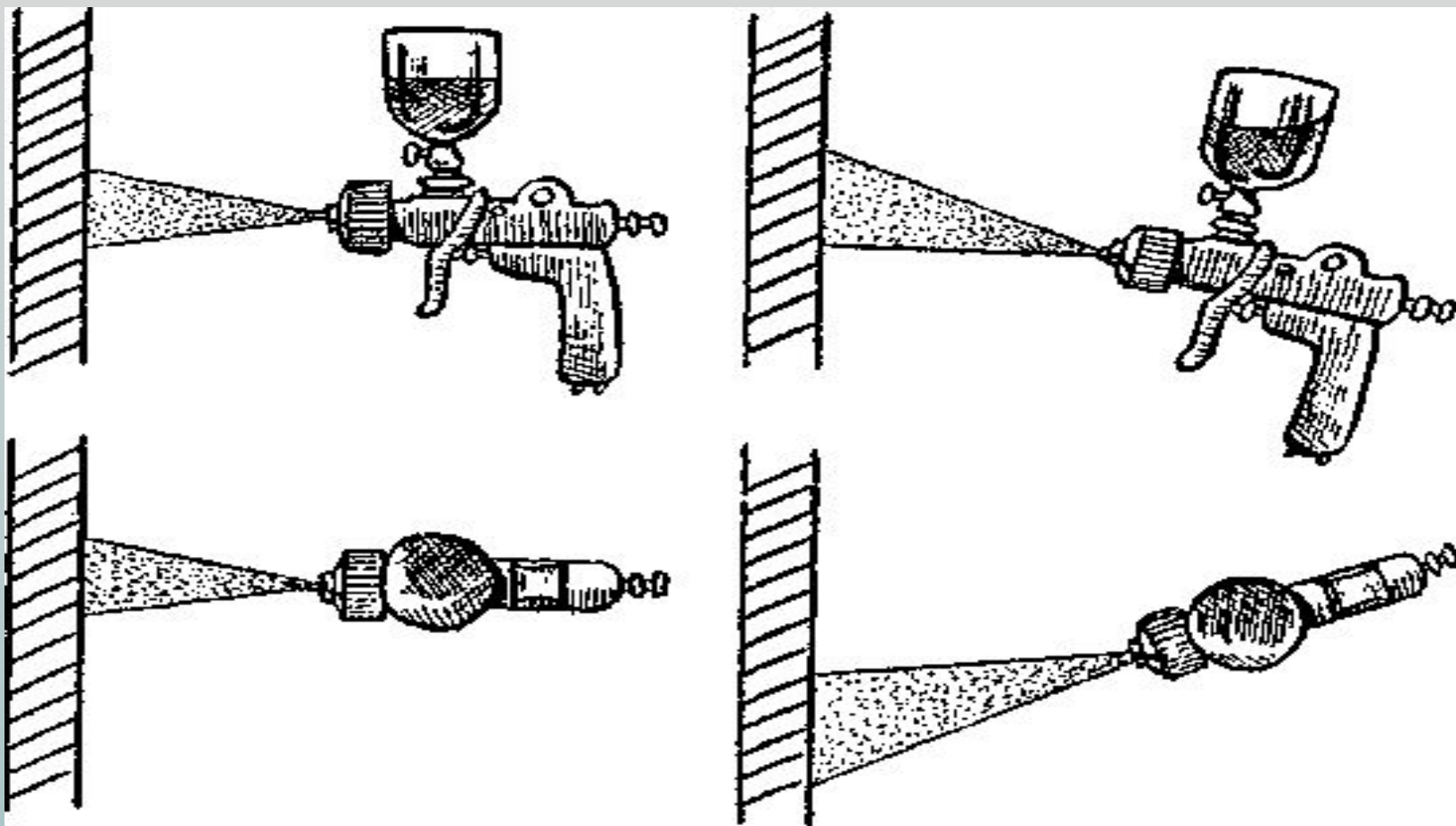
Рис. 45. Положение пульверизатора во время окрашивания а — правильно; б — неправильно
