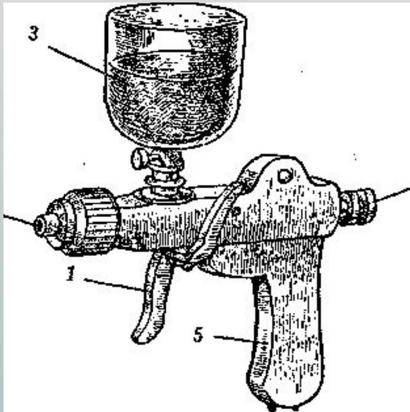
•Рис. 44. Пульверизатор: 1 — курок; 2 - сопло; 3 - емкость для краски-4 — регулятор поршня; 5 — трубка для подачи воздуха
