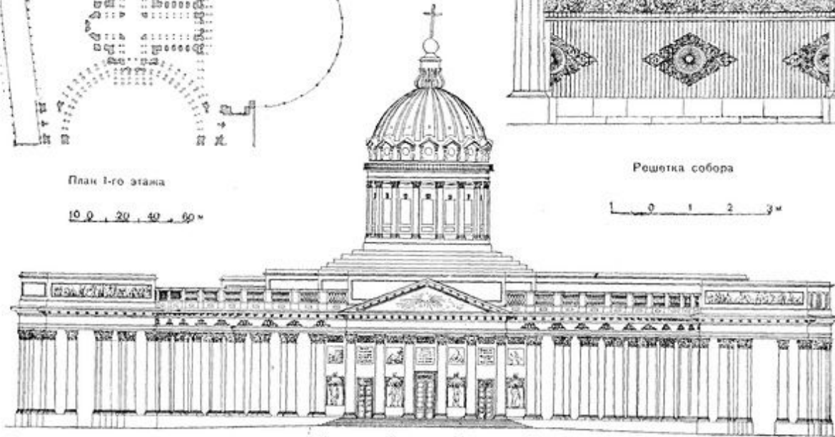
Северный фасад
