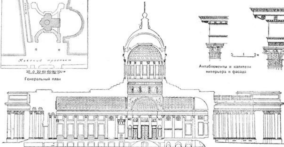
Продольный разрез
