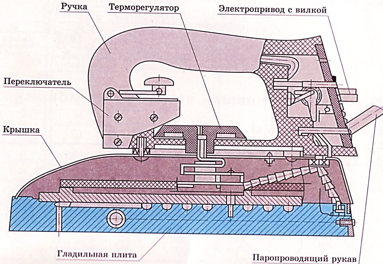
Схема утюга
