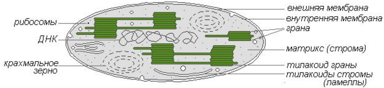
Строение хлоропласта
