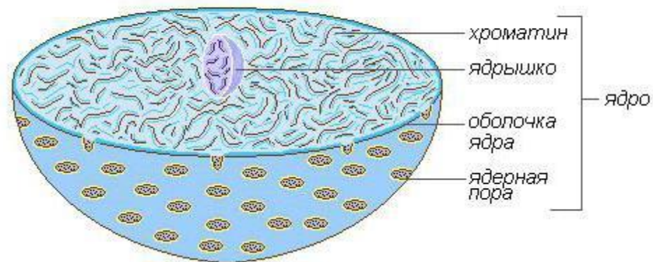
Строение ядра
