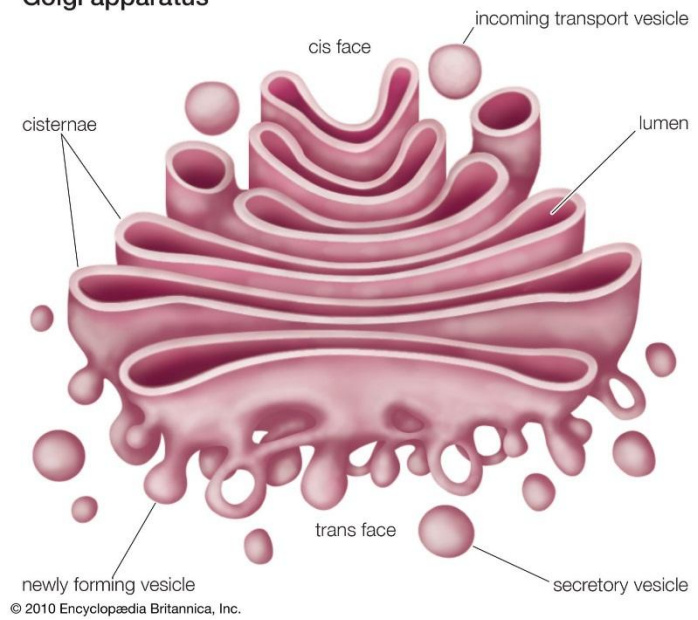
Golgi apparatus
