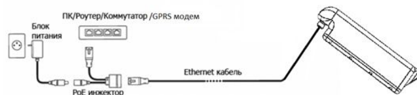
Схема подключения:
