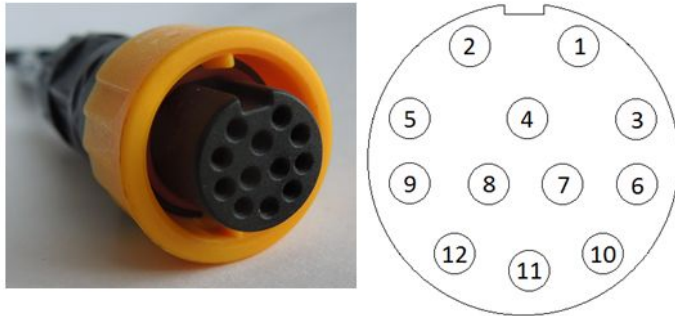
Схема разъема кабеля ДСПД
