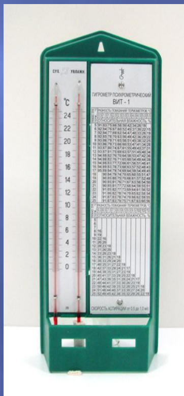
ПСИХОМЕТР
