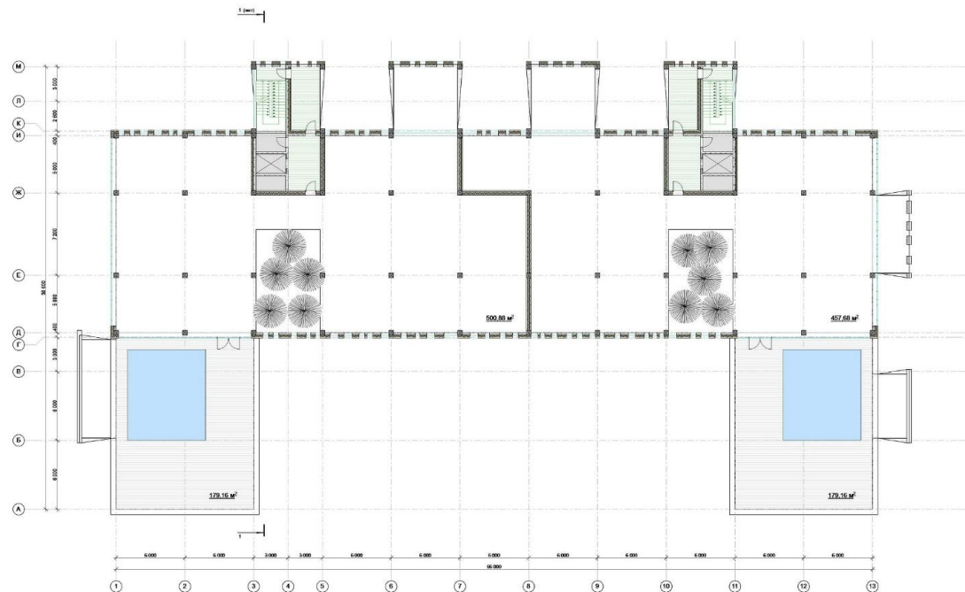
План 17 этажа
