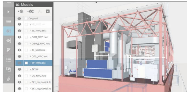
Сводная модель в BIM 360 Glue. Изображение предоставлено ООО «РОСЭКО-СТРОЙПРОЕКТ»
