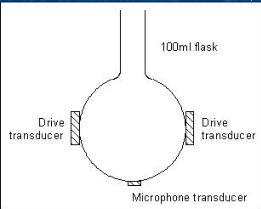
Схема установки
