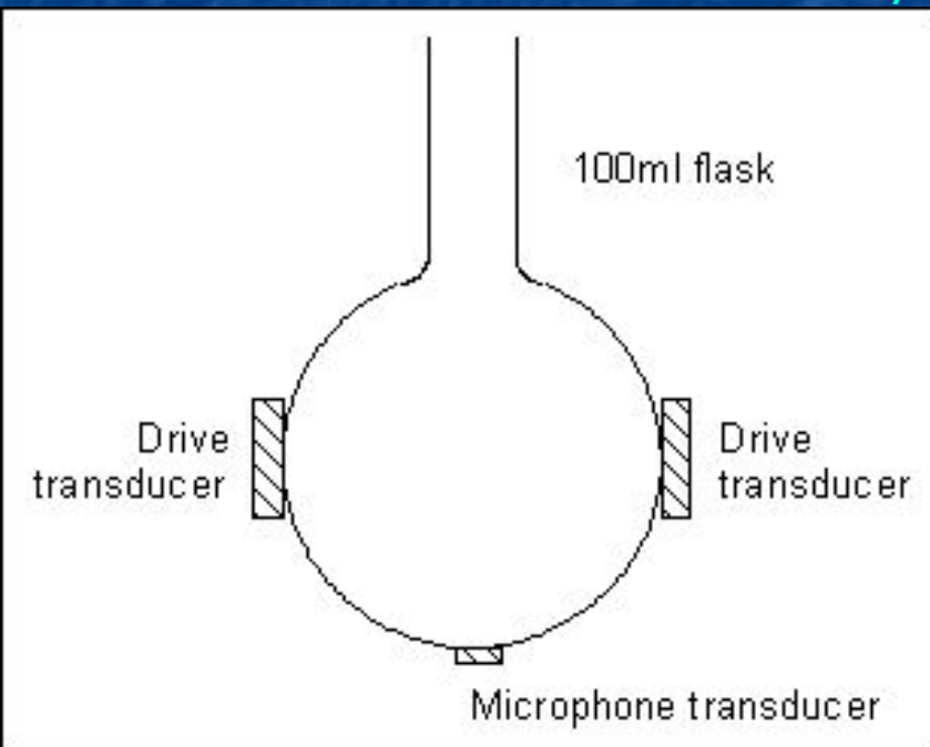
Схема установки
