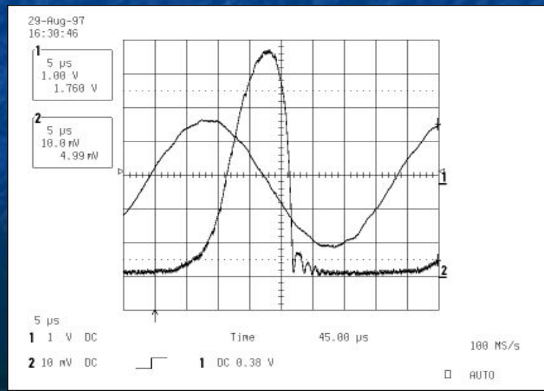
Акустическое давление и радиус пузырька в зависимости от времени
