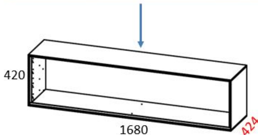
TUM-926/*** Тумба TB VERSO 420x424 (каркас)
