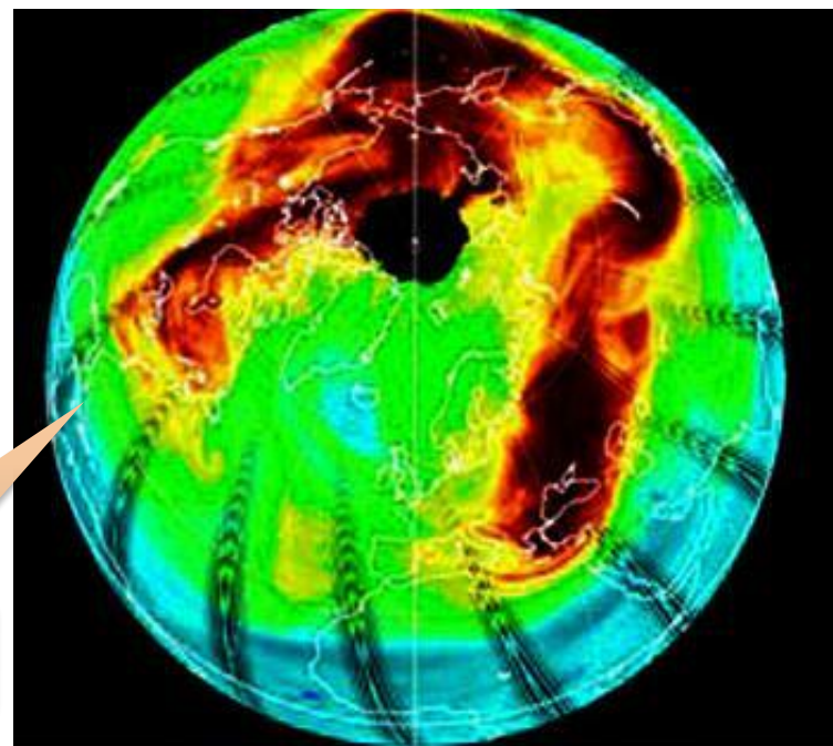
<100 180 260 340 420 500> Ozone (Dobson Units)
