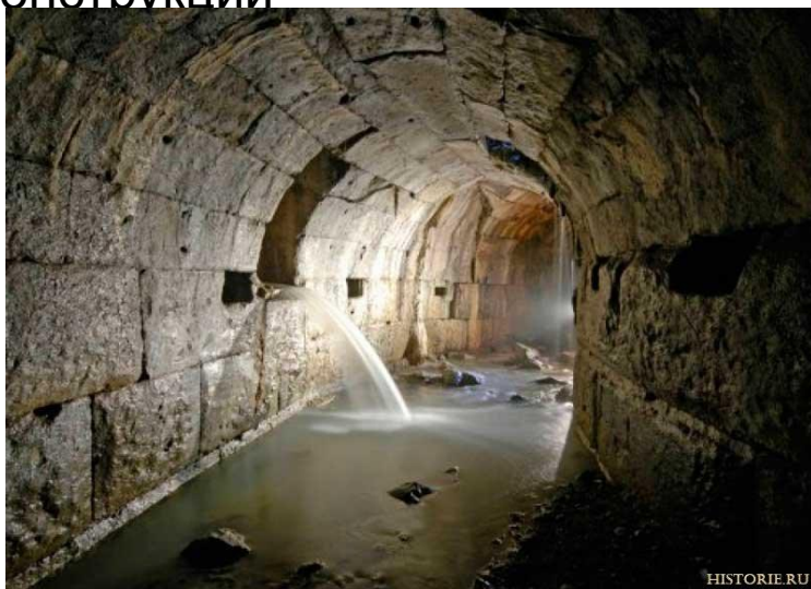
Акведук Аппия Клавдия 311 до н.э и примерная схема КОНСТРУКЦИИ
