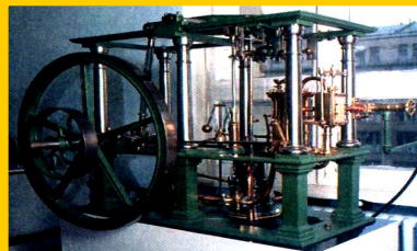
Паровая машина Дж.Уатта. Современная модель
