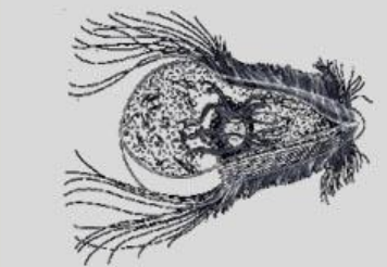
Trichonympha collaris из задней кишки термитов и древесных тараканов. (о. HYPERMASTIGINA)
