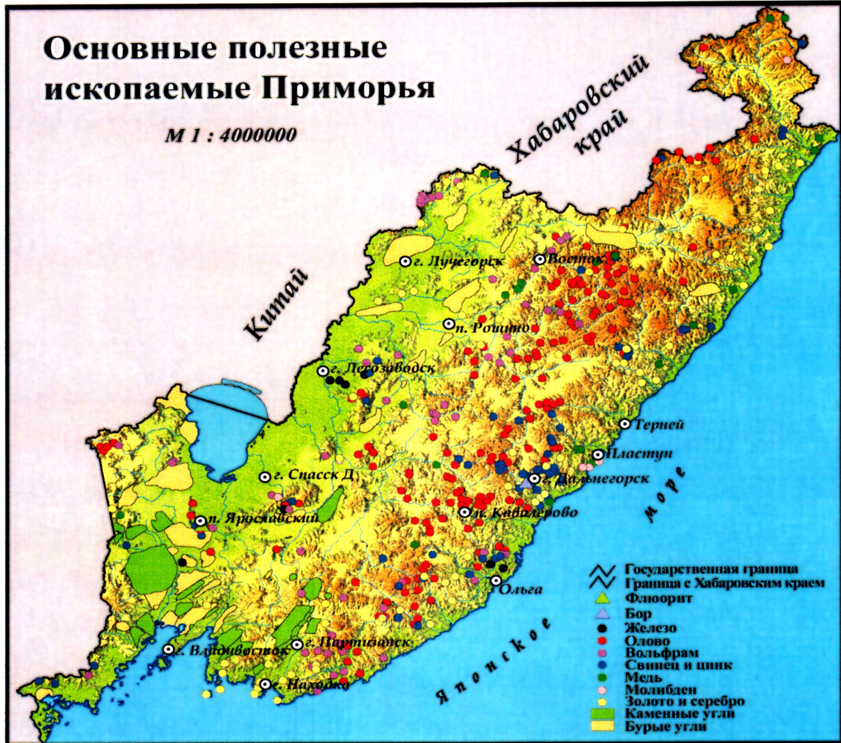
Карта месторождений основных полезных ископаемых Приморского края
