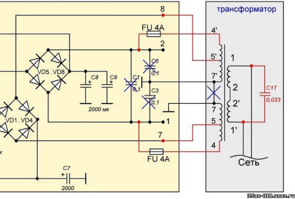
U3 Плата выпрямителя
