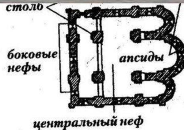
Крестово-купольный храм
