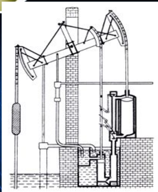
Схема паровой машины Д. Уатта (1775 г.)
