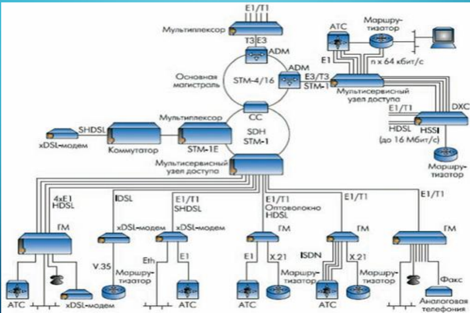
РИС. 2. Современный вариант организации сети доступа
