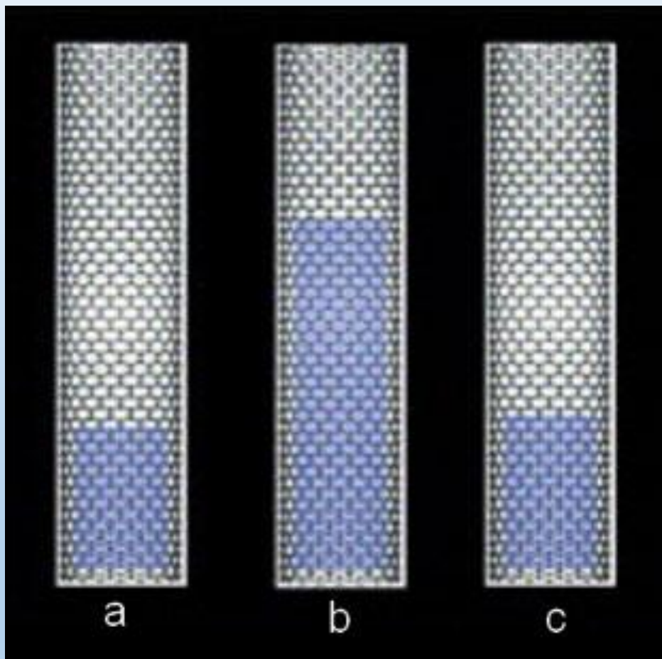
Углеродный нанотермометр, наполненный Ga, показывающий расширение Ga внутри CNT при температурах (a) 58°C, (b) 490°C, и (c) 45°C.
