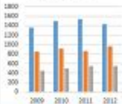
Гистограмма
