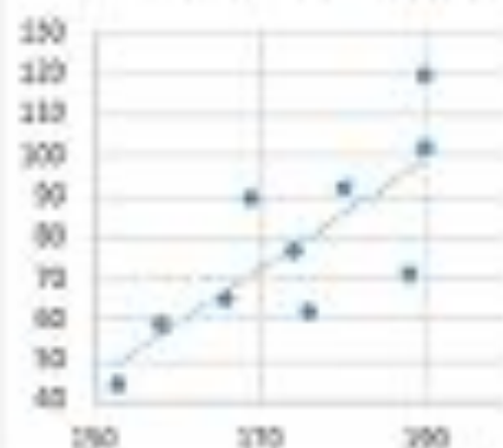
Точечная диаграмма
