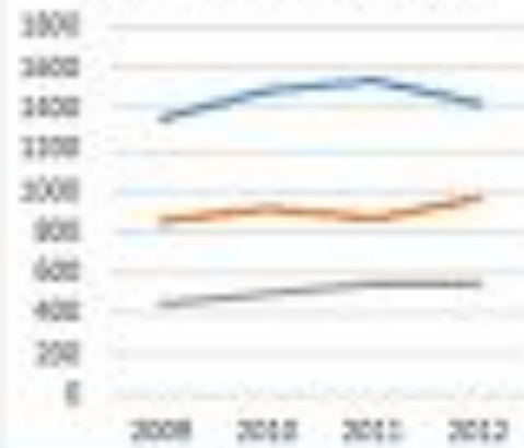
Линейный график
