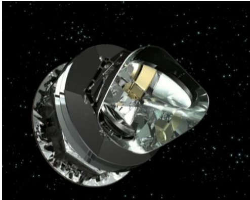
Космическая обсерватория Планк Карта анизотропии реликтового излучения
