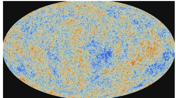
Космическая обсерватория Планк Карта анизотропии реликтового излучения
