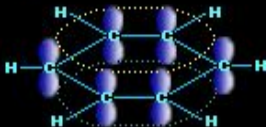
Делокализация \pi -электронов
