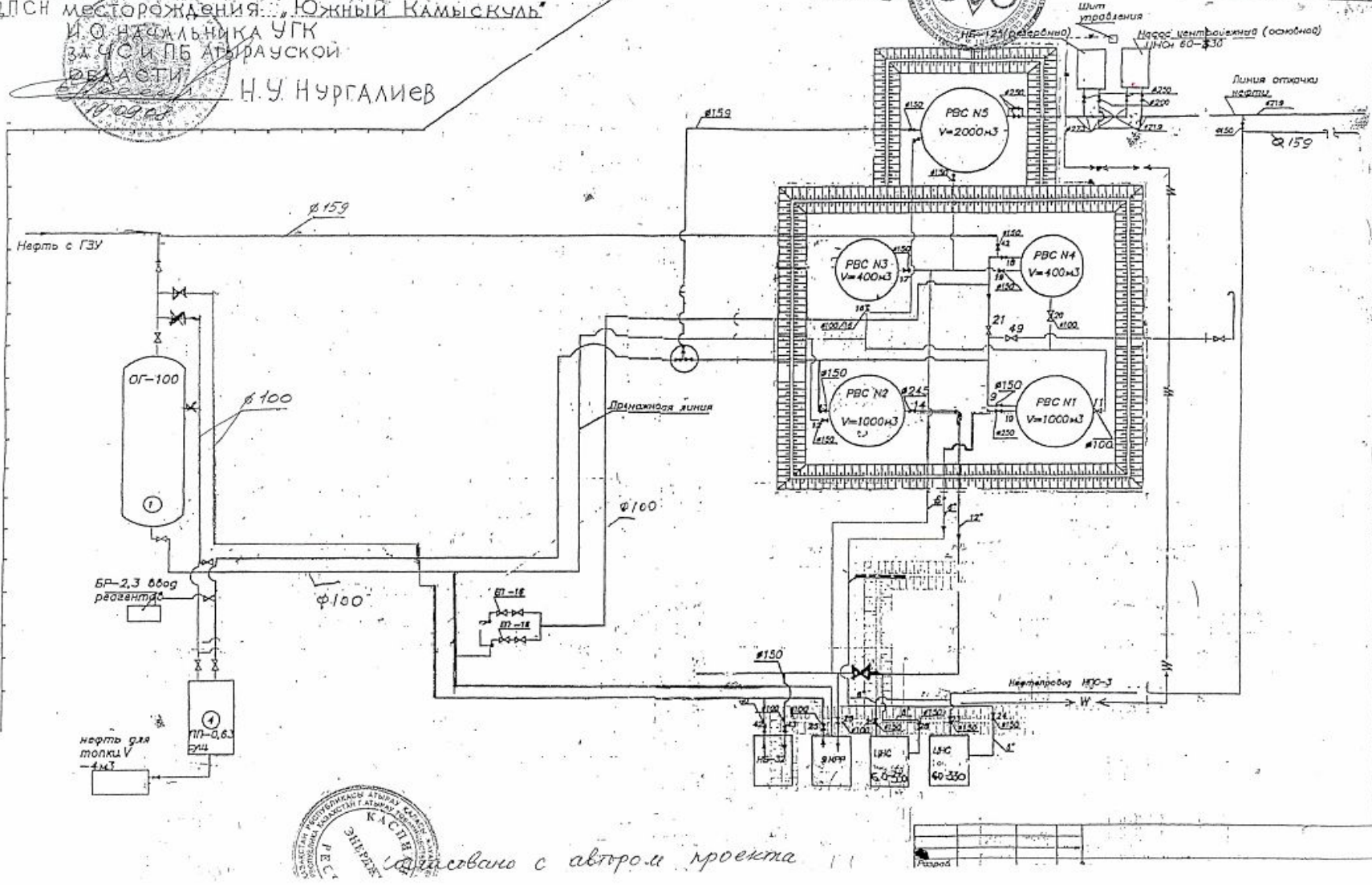
● Мұнайды жинау орталық пунктiнiң технологиялық схемасы
