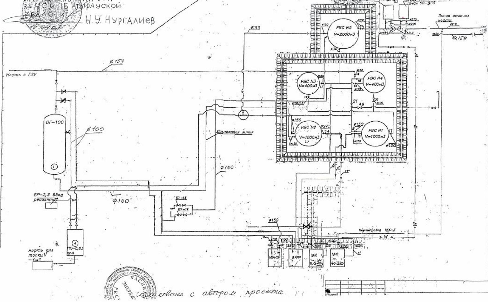
● Мұнайды жинау орталық пунктiнiң технологиялық схемасы
