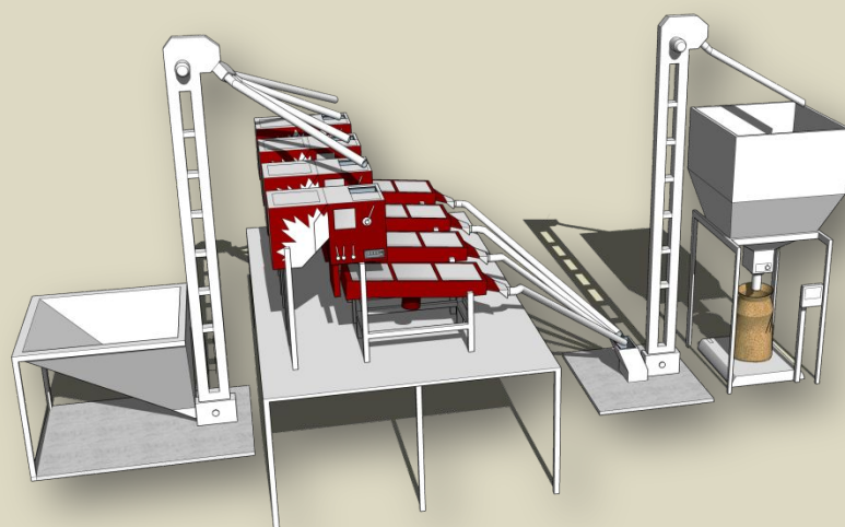
Поточные зерноочистительные линии на базе машин АРЗМ-КЛЕН
