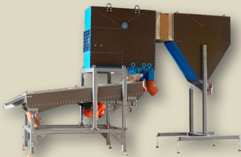
Зерноочистительная машина АРЗМ-КЛЕН 2
