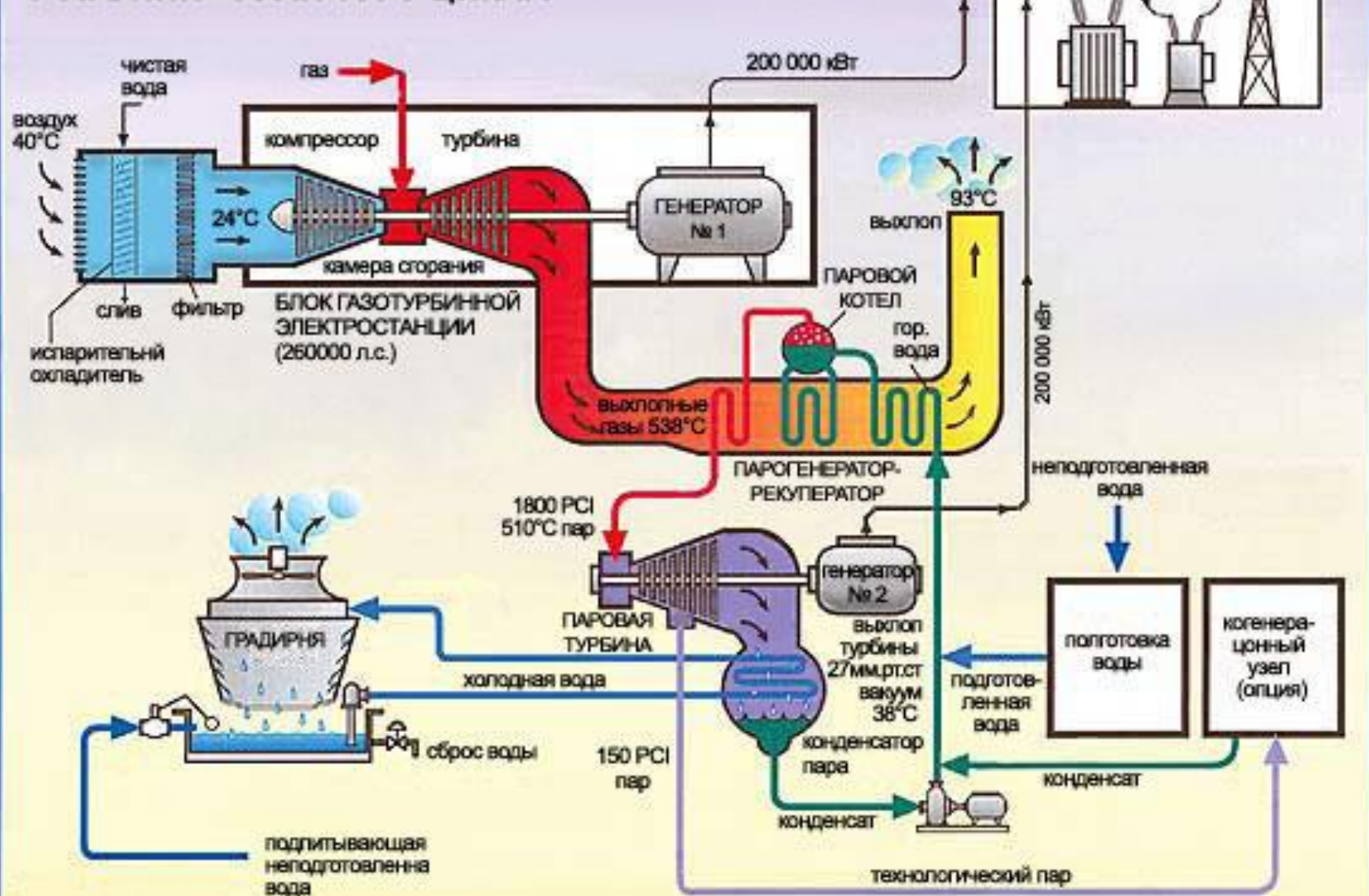
СХЕМА ГАЗОТУРБИНОЙ ЭЛЕКТРОСТАНЦИИ КОМБИНИРОВАННОГО ЦИКЛА
